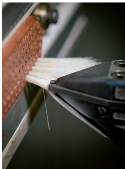
Ci dessous: Le pinceau de poil a été poinçonné dans le corps de brosse.
